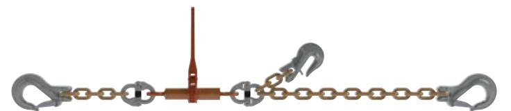
1-teilige Zurrkette 16-10 mit DoRa200 1-piece lashing chain 16-10 with DoRa200
