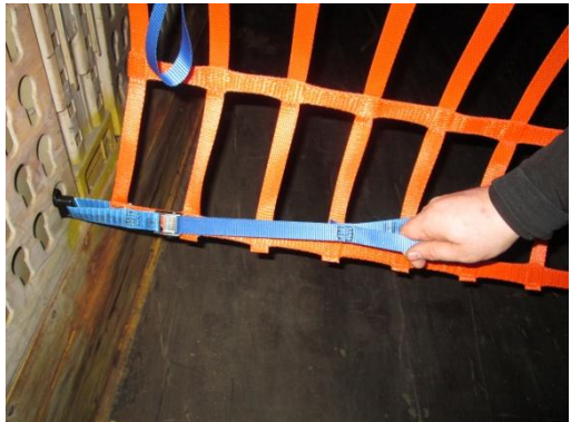
Abb. 15: Die drei Spannelemente mit Hilfe der Handschleife anziehen. Anschließend ist die Ladung Rückwärtig normkonform gesichert
