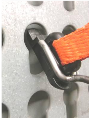
Abb. 12-13: Für den Überkopfeinsatz kann die Montagehilfe verwendet werden. Dazu Fitting auf die Montagehilfe stecken.
